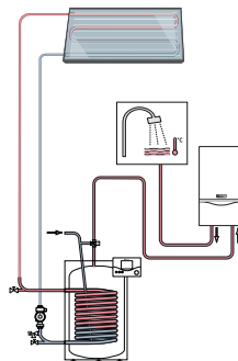
auroSTEP plus 150 + ecoTEC plus VCW
